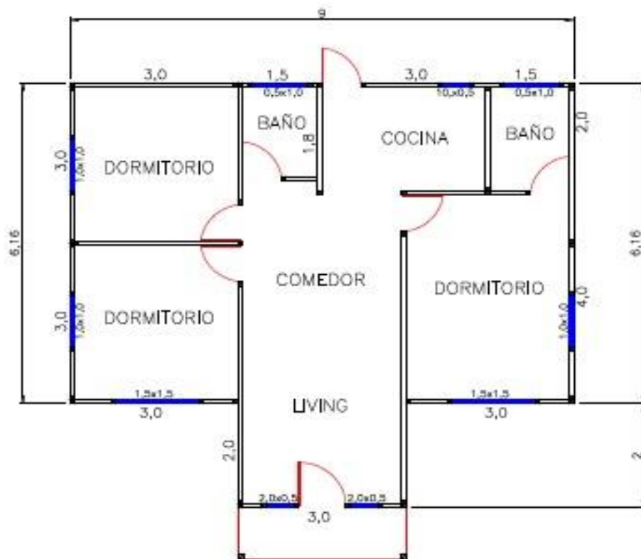
PLANTA DISTRIBUCION MODELO VILLARRICA 63mts. 2
